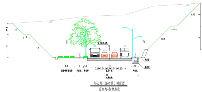
富兴路至加林路横断面图
