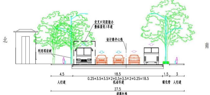
北三路横断面图
