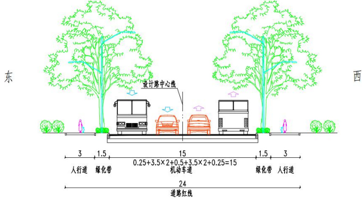
环山路标准横断面图
