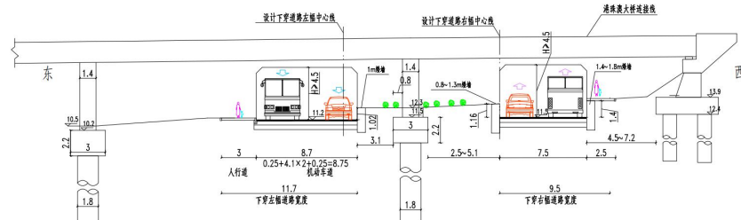
下穿港珠澳大桥连接线横断面图
