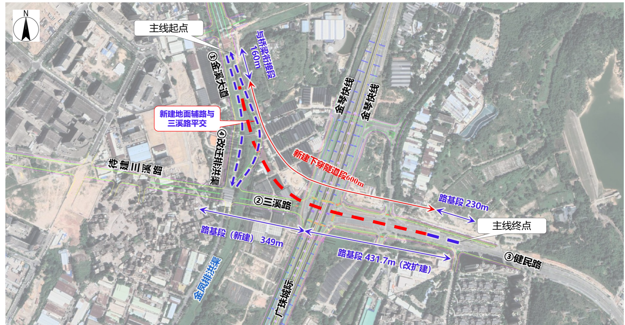
金溪大道下穿金琴快线隧道工程线位图
