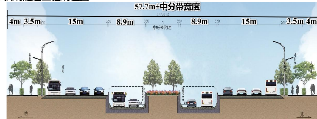
隧道健民路端敞口段横断面图
